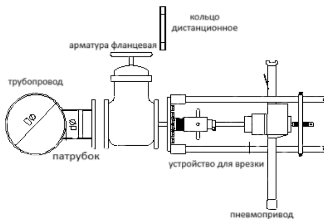
Схема подключения к трубопроводу через фланцевое соединение
